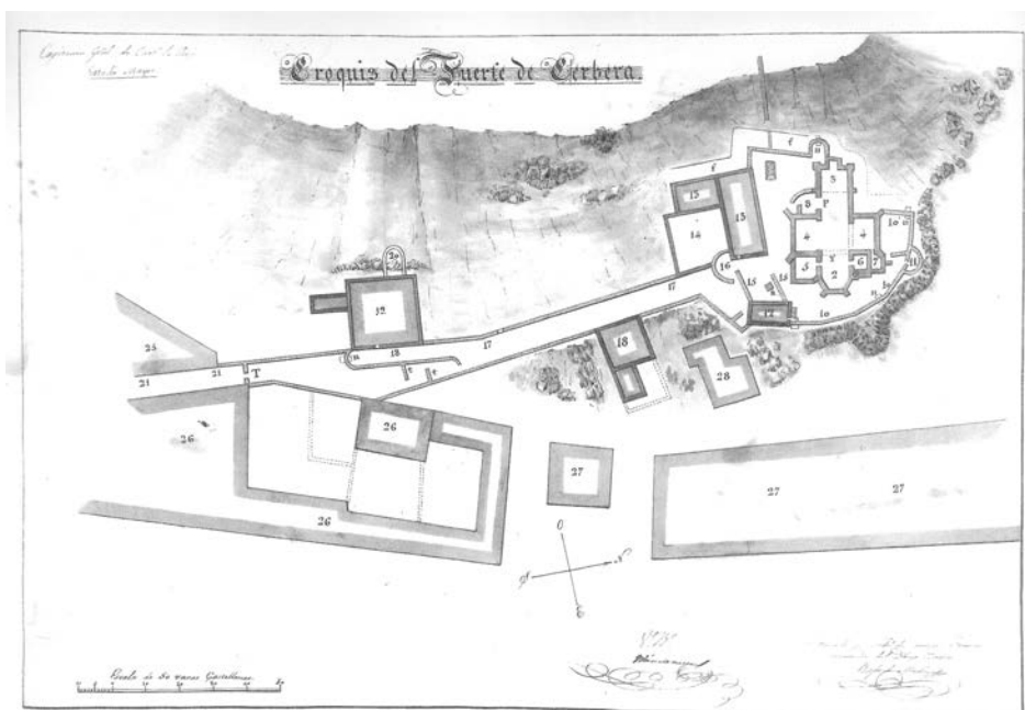
Fig. 1. Croquis del Fuerte de Cervera realizado por el capitán de Cuerpos Francos D. Rafael Medina en 1838.
